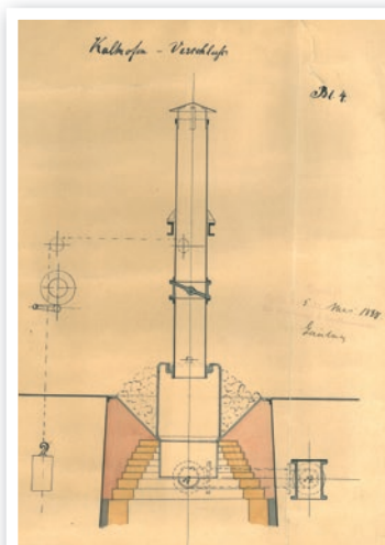
Bauzeichnung des Kalkofens von 1898.
