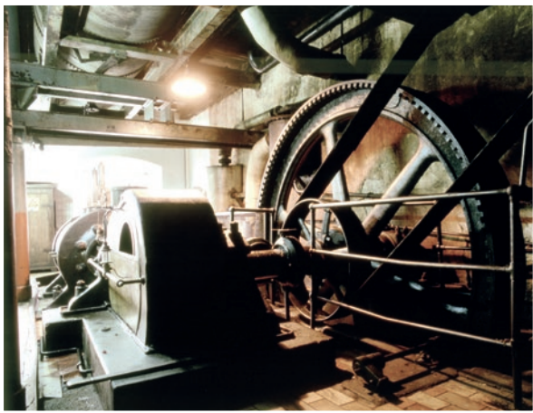
Liegende Einzylinder-Dampfmaschine, die über Schwungrad mit Riemenscheibe und Transmissionssystem die Rührwerke – früher auch die Zentrifugen – antreibt. Hersteller: Braunschweigische Maschinenbauanstalt; Baujahr 1921, Leistung 88 kW (120 PS), Dampfverbrauch 1,5 t/h, Schwungrad mit 3.500 mm Durchmesser, Drehzahl 100 min -1 .
