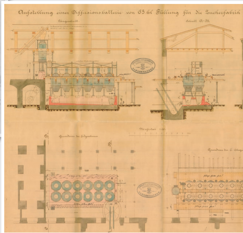
Diffusionsbatterie-Anlage.
