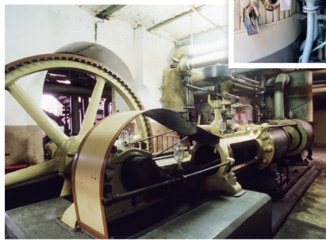
Liegende Einzylinder-Dampfmaschine mit Schiebersteuerung (1918) in sehr langer Bauweise: eine Kolbenstange für Dampf- und Pumpenzylinder.
