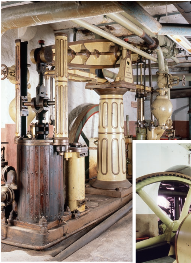
Balancier-Dampfmaschine (1882), Hersteller Maschinenfabrik Sangerhausen, mit Schwungrad 2.700 mm Durchmesser, Drehzahl 25–30 min -1 , für den Antrieb der Kalkmilchpumpe.
